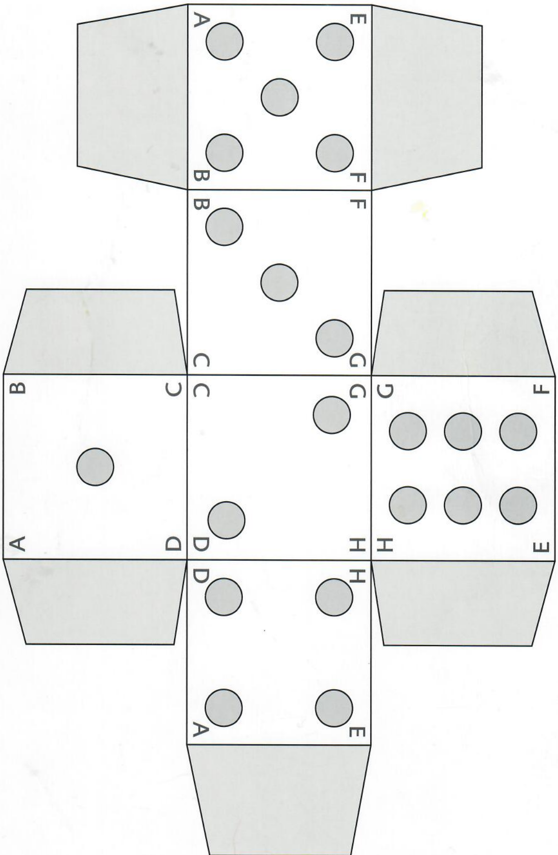
Faltnetz eines Würfels
